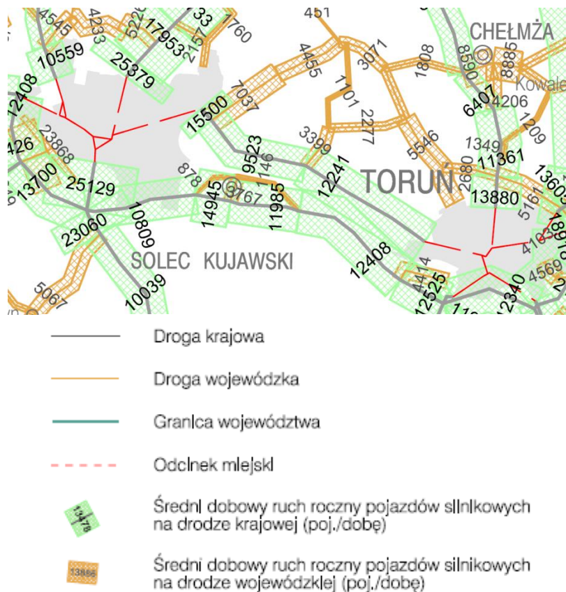
Rysunek 24. Średni dobowy ruch roczny pojazdów silnikowych na sieci dróg krajowych i wojewódzkich w 2015 roku
