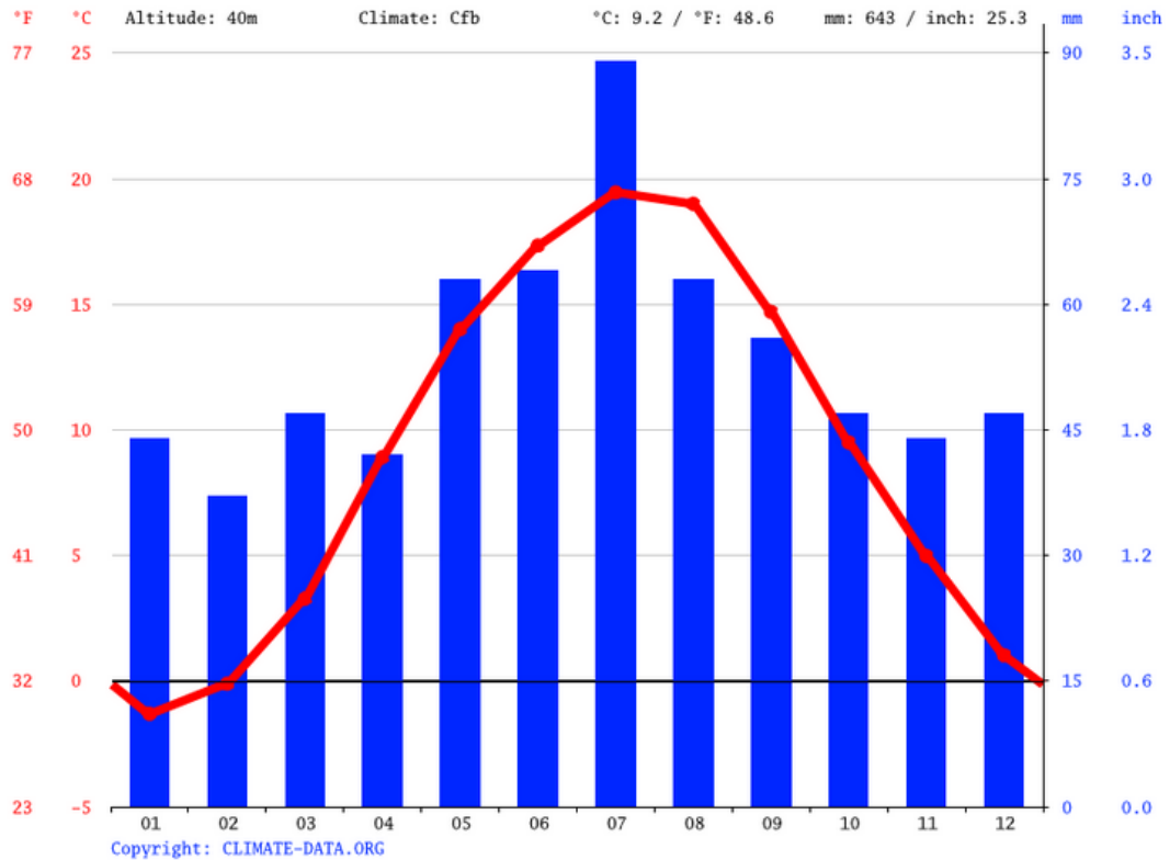
Rysunek 18. Klimatogram dla miejscowości Górsk Źródło: opracowanie własne na podstawie www.climate-data.org
