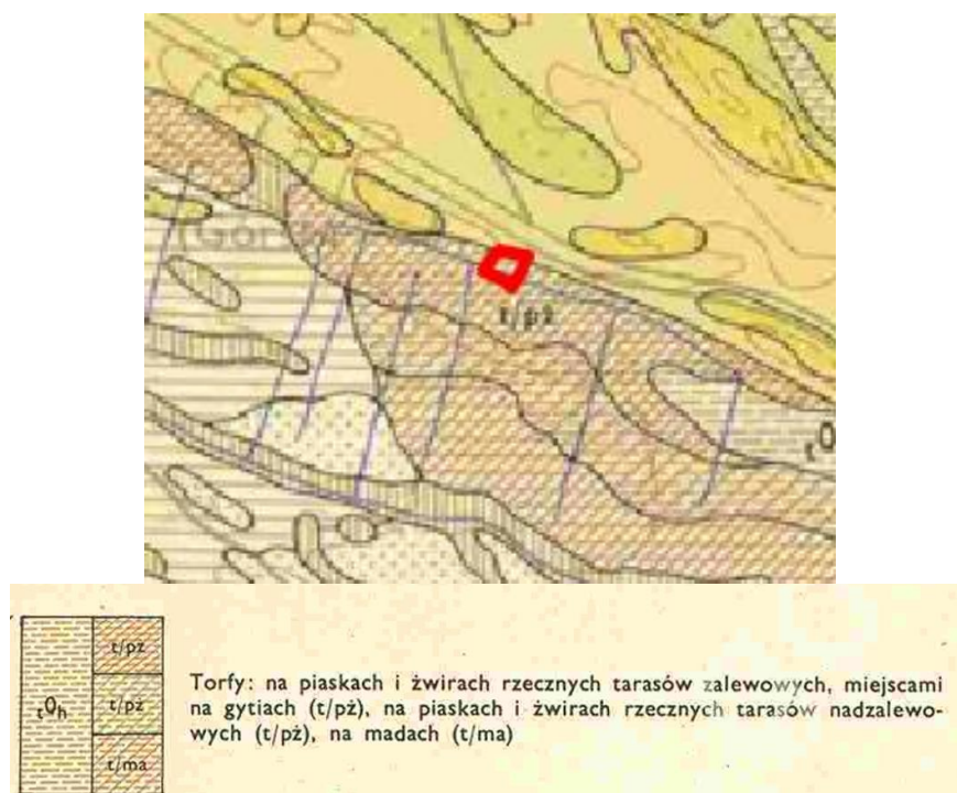
Rysunek 8. Szczegółowa Mapa Geologiczna Polski 1:50 000 wraz z zaznaczonym obszarem opracowania Źródło: Szczegółowa Mapa Geologiczna Polski 1:50 000 Arkusz Rzęczkowo 320
