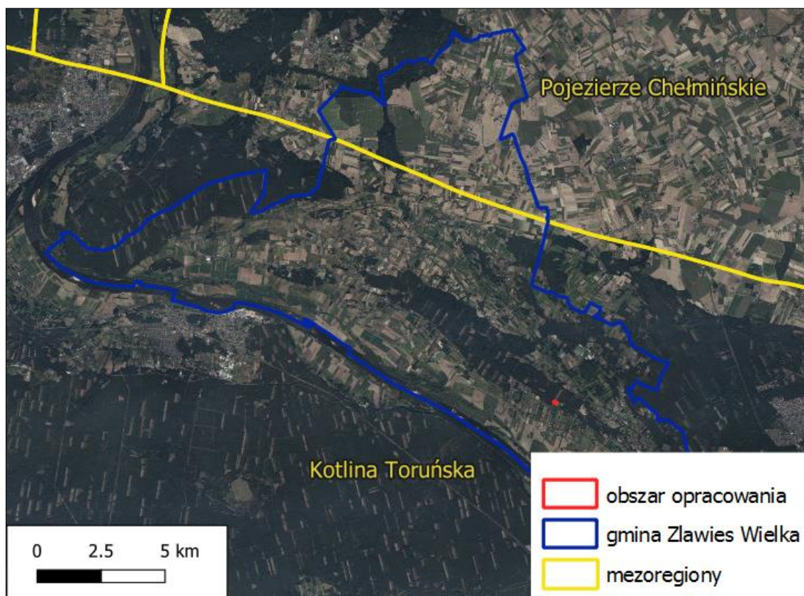
Rysunek 6. Regiony fizyczno-geograficzne na terenie obszaru opracowania Źródło: opracowanie własne
