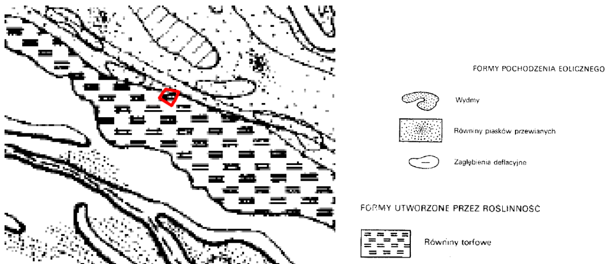
Rysunek 7. Fragment Szkicu Geomorfologicznego Polski 1:50 000 wraz z zaznaczonym obszarem opracowania Źródło: Objasnienia do Szczegółowej Mapy Geologicznej Polski w skali 1:50 000 Arkusz Rzęczkowo 320
