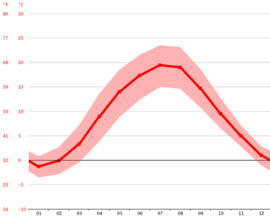
Rysunek 19. Wykres temperaturowy dla miejscowości Górsk Źródło: opracowanie własne na podstawie www.climate-data.org
